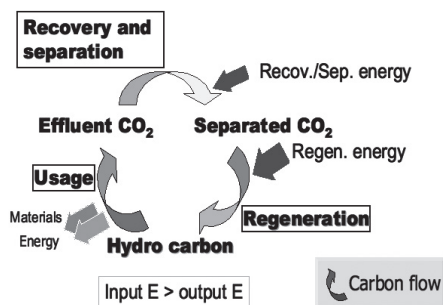
図3 能動的な炭素循環型エネルギーシステム (ACRES) の基本構成
